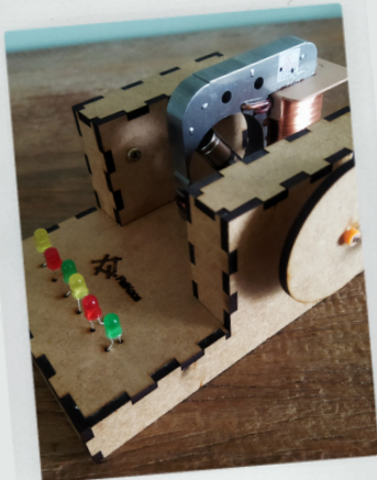
GERADOR DE ELETRICIDADE
