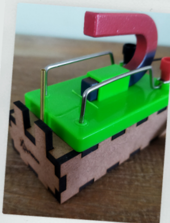
FORÇA MAGNÉTICA
